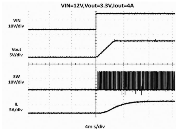
Fig 29. Vin Power On
