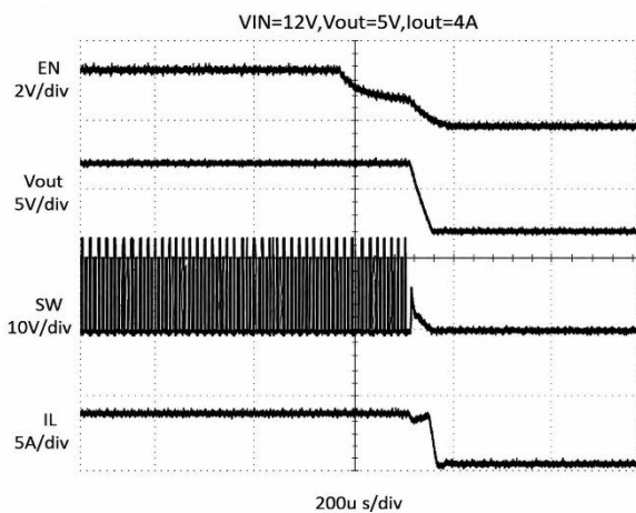
Fig 35. EN OFF
